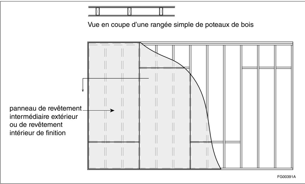
Figure A-9.10.3.1-F Application verticale du revêtement intermédiaire d'un mur extérieur ou du revêtement de finition d'un mur intérieur, tous les joints étant supportés par des éléments en bois de construction de mêmes dimensions que celles des éléments d'ossature (1) La figure est fournie à des fins explicatives seulement et n'est pas à l'échelle.
