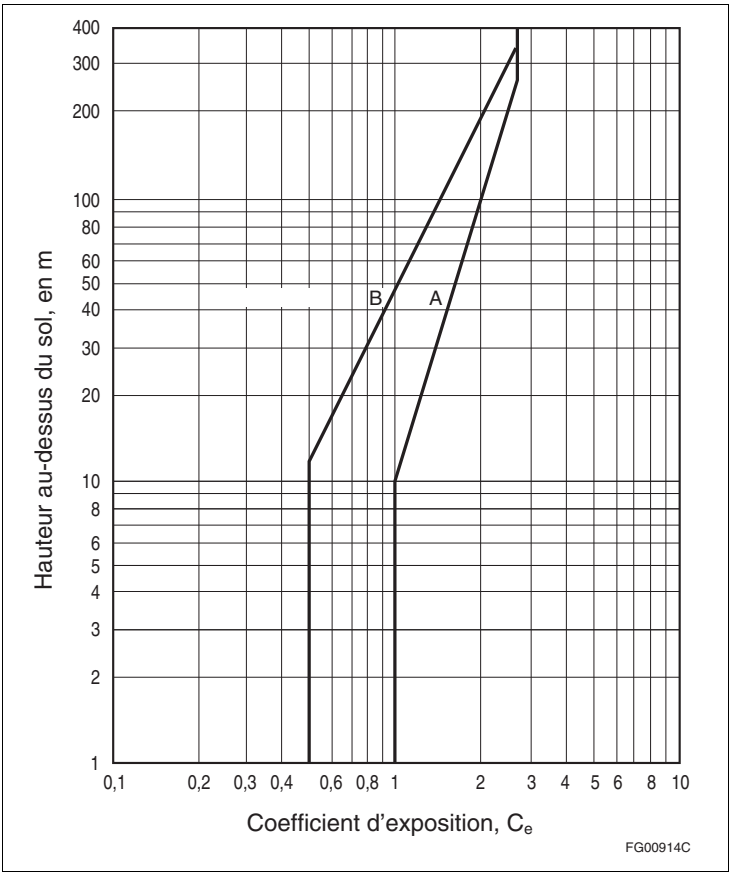
Figure A-4.1.7.8. 2) et 3) Coefficient d'exposition, C_e , pour la méthode dynamique (1) La courbe A représente C_e pour un terrain à découvert tel que défini à l'alinéa 4.1.7.3. 5)a). (2) La courbe B représente C_e pour un terrain rugueux tel que défini à l'alinéa 4.1.7.3. 5)b).
