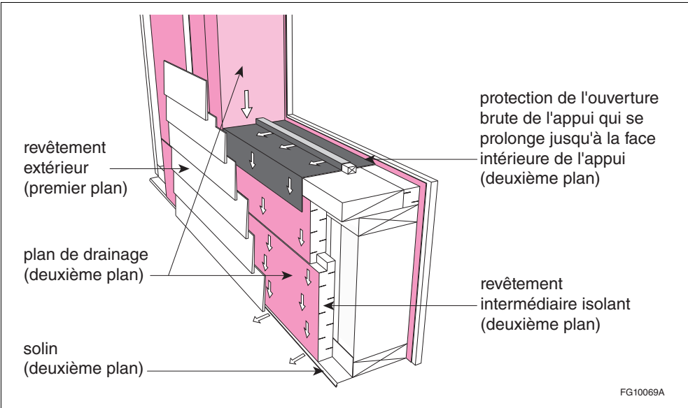
Figure A-9.27.2-C Mur de protection contre la pluie avec un deuxième plan de protection composé d'un revêtement isolant
