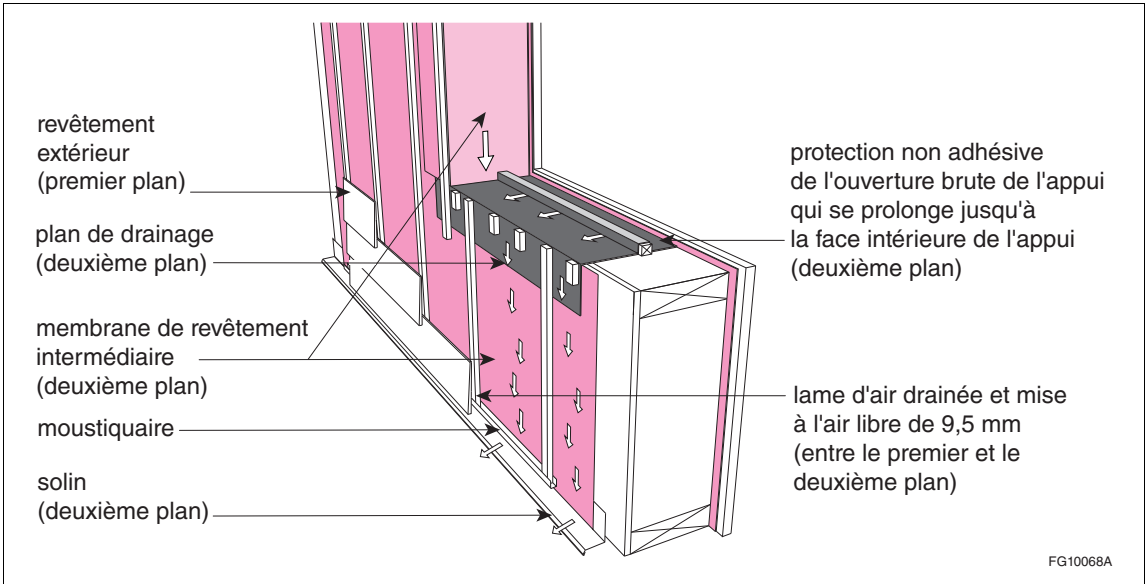
Figure A-9.27.2-B Mur de protection contre la pluie avec un deuxième plan de protection composé d'un système de lame d'air mise à l'air libre et drainée
