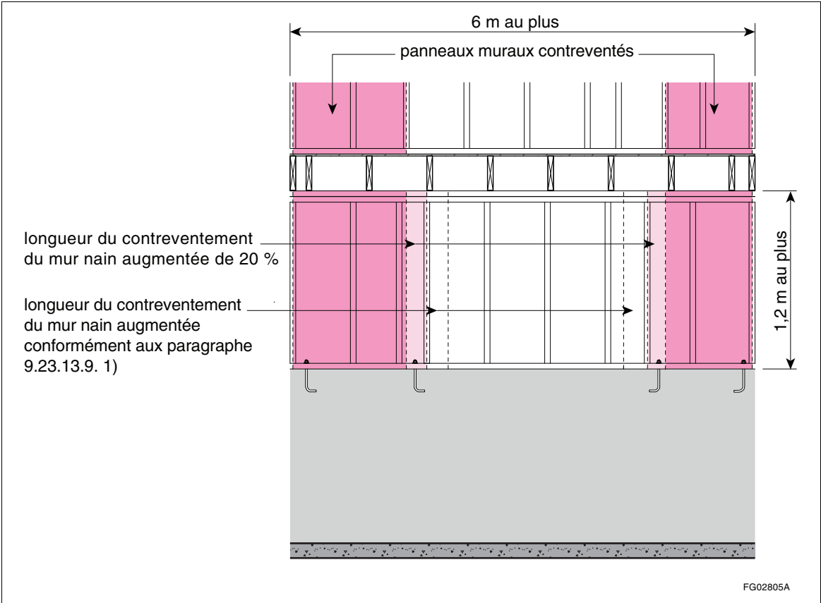
Figure A-9.23.13.10. 2) Mur nain de fondation si S_{\max} \leq 0,60
