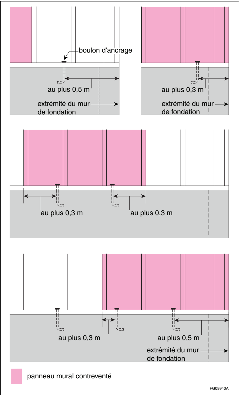
Figure A-9.23.6.1. 3) Ancrage des panneaux muraux contreventés
