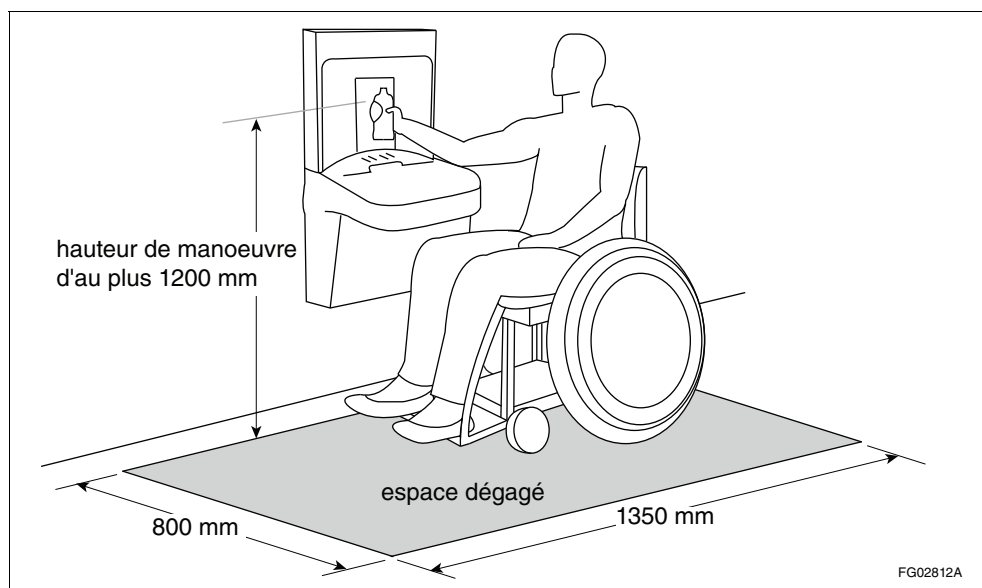
Figure A-3.8.3.11. 2)b) et d) Espace dégagé et hauteur de manœuvre exigés pour les stations de remplissage de bouteilles d'eau
