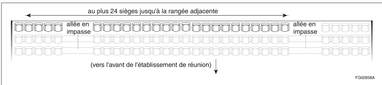
Figure A-3.3.2.5. 5) Calcul des 24 sièges jusqu'à une autre allée
