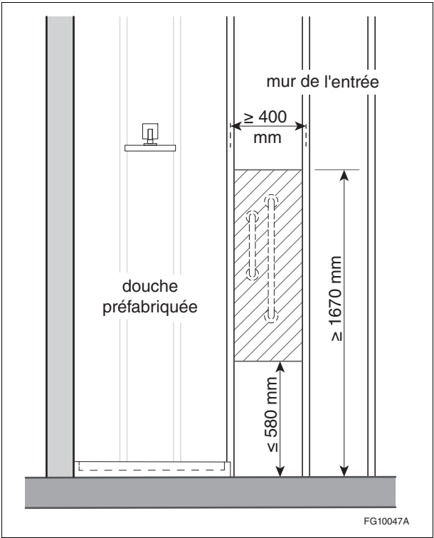
Figure A-3.8.4.4. 5)-A Exemple d'une configuration acceptable pour le renforcement du mur de l'entrée d'une douche munie d'une cabine préfabriquée
