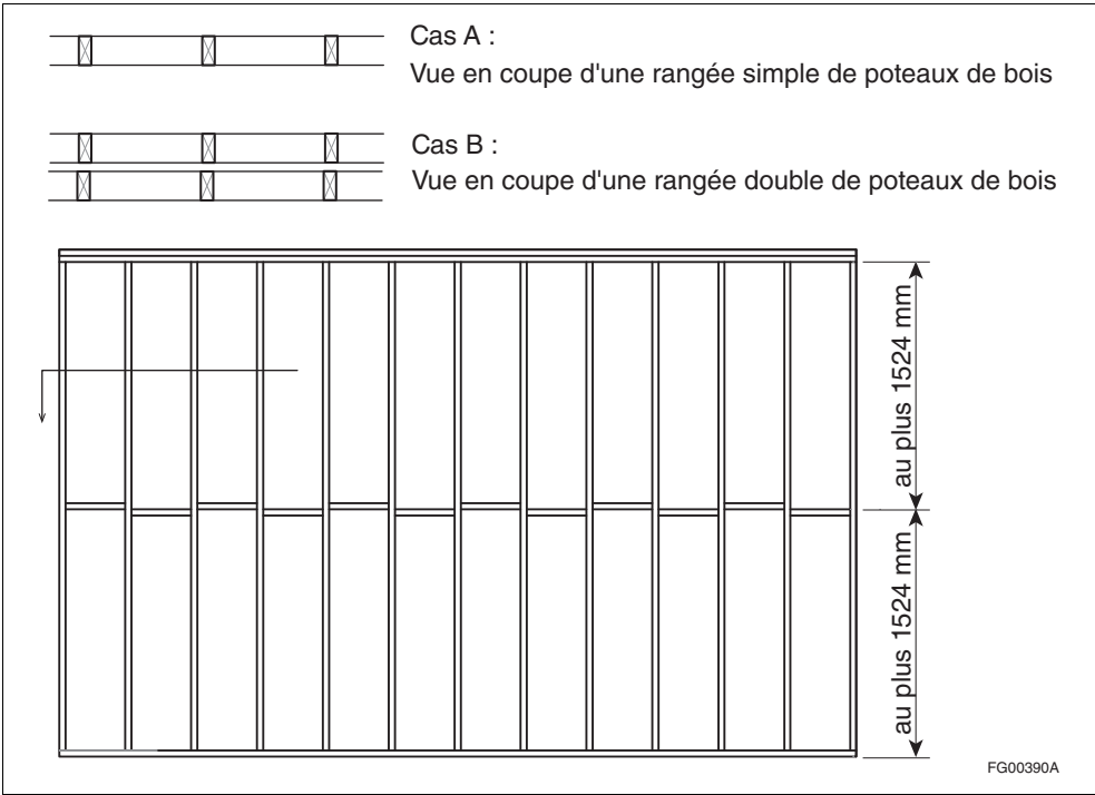
Figure A-9.10.3.1-E Cales destinées à des murs à ossature de bois légère comprenant une rangée simple ou double de poteaux (1) La figure est fournie à des fins explicatives seulement et n'est pas à l'échelle.
