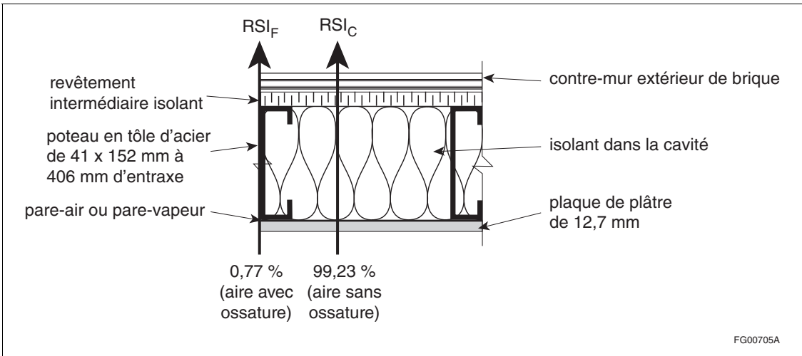
Figure 2-1 Paramètres de calcul de la valeur RSI_{eff} pour un mur à ossature en tôle d'acier de 41 × 152 mm
