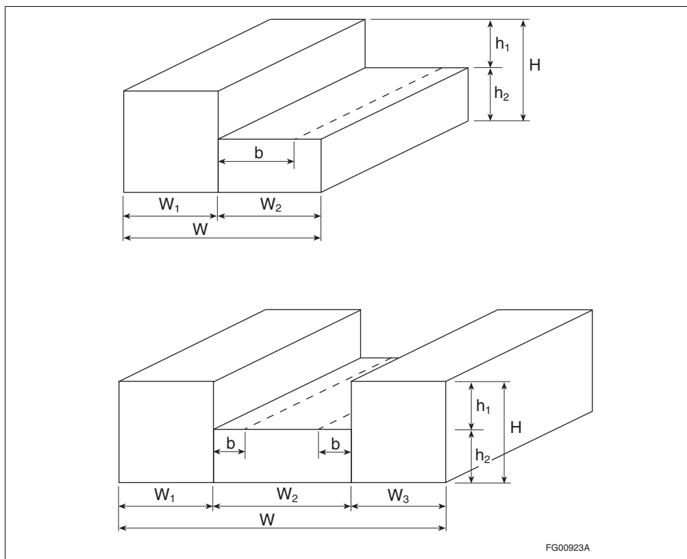
Figure 4.1.7.6.-D Valeurs extérieures de pointe du produit C_g C_p pour le calcul des composants structuraux et du revêtement extérieur des bâtiments à toiture-terrasse en gradins Faisant partie intégrante du paragraphe 4.1.7.6. 5)
