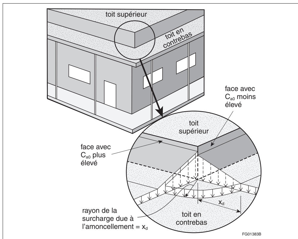
Figure 4.1.6.8.-B Charge due à la neige au coin intérieur Faisant partie intégrante du paragraphe 4.1.6.8. 2)
