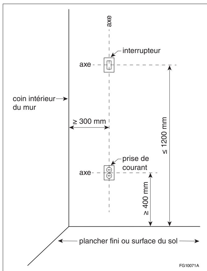
Figure A-3.8.4.2. 1) Position des axes des interrupteurs et des prises de courant
